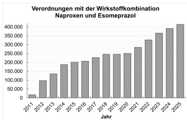
Abbildung: Mit der sozialen Krankenversicherung österreichweit abgerechnete Präparate mit der Wirkstoffkombination Naproxen und Esomeprazol (ATC-Code M01AE52) vom Jahr 2011 bis zum Jahr 2025 3
